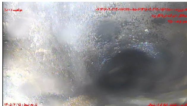
شماره تصویر ۲ عنوان تراز آب / تراز آب کدر موقعیت ۱۰۰ کد WLT ۵ درصد
