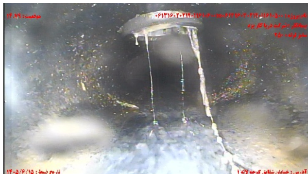
شماره تصویر ۷ عنوان اتصال جانبی معيوب/اتصال معيوب انشعاب موقعیت ۱۴.۷۹ کد CX
