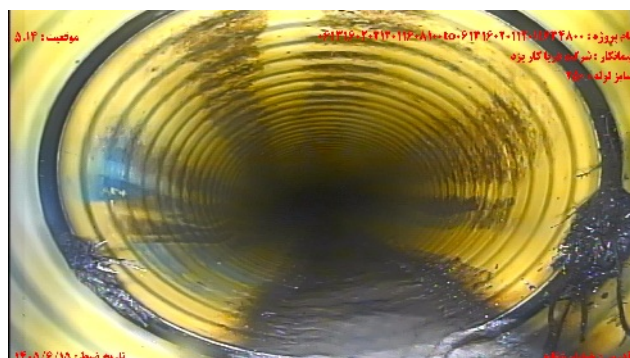
شماره تصویر ۴ عنوان نفوذ ریشه / نفوذ انبوه ریشه ها و گاهی سطح مقطع به میزان % موقعیت ۵۰۱۴ کد RM درصد ۱۰
