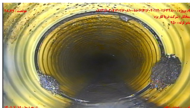
شماره تصویر ۶ عنوان نفوذ ریشه / نفوذ انبوه ریشه ها و گاهی سطح مقطع به میزان % موقعیت ۲۸۰۳۷ کد RM درصد ۱۰
