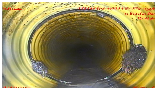
شماره تصویر ۵ عنوان اتصال باز / به میزان % قطر موقعیت ۲۸۰۳۷ کد OJ
