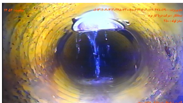
شماره تصویر ۳ عنوان موقعیت ۱۳-۵۳ کد محل اتصال انشعاب / اتصال انشعاب CN
