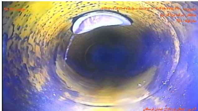
شماره تصویر: ۷ موقعیت: ۲۸.۱۶ کد: CN عنوان: محل اتصال انشعاب / اتصال انشعاب
