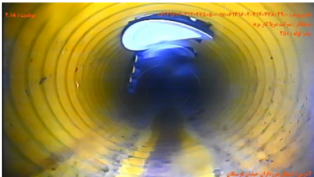
شماره تصویر ۳ عنوان اتصال جانبی معيوب /اتصال معيوب انشعاب
