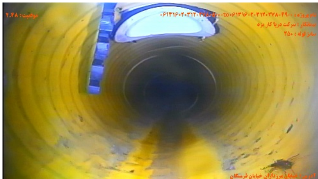
شماره تصویر ۴ عنوان محل اتصال انشعاب /اتصال انشعاب
