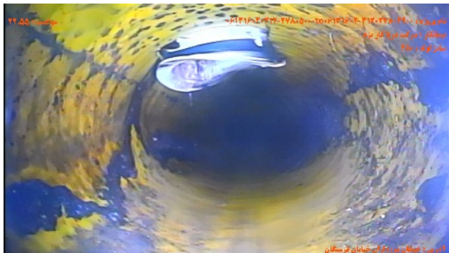
شماره تصویر ۶ عنوان اتصال جانبی معيوب /اتصال معيوب انشعاب
