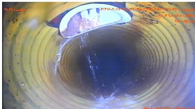
شماره تصویر ۷ عنوان محل اتصال انشعاب / اتصال انشعاب موقعیت ۲۹.۲۶ کد CN
