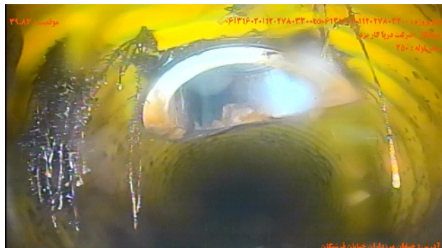
شماره تصویر ۱۳ موقعیت ۳۹.۸۳ کد CX عنوان اتصال جانبی معيوب/اتصال معيوب انشعاب
