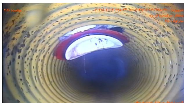
شماره تصویر ۳ عنوان موقعیت ۲.۹۰ کد CX اتصال جانبی معيوب / اتصال معيوب انشعاب
